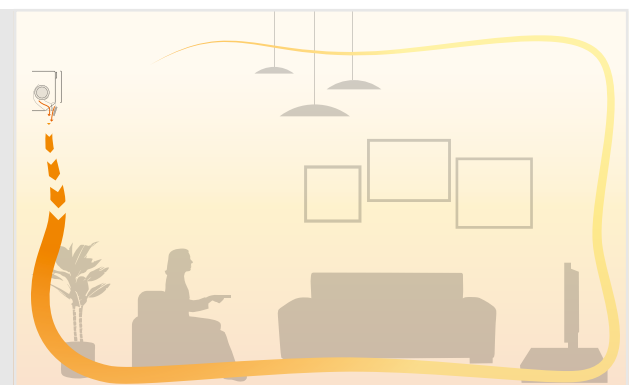
Het Coanda-effect creëert twee verschillende luchtstroompatronen afhankelijk van of koel- of verwarmingsfunctie is geactiveerd. De bovenste afbeeldingen tonen het Coanda-effect in koelmodus (plafondluchtstroom) en de onderste in verwarmingsmodus (verticale luchtstroom).
